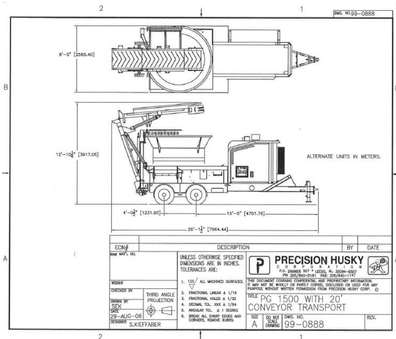
图 1-5 破碎機外形圖
