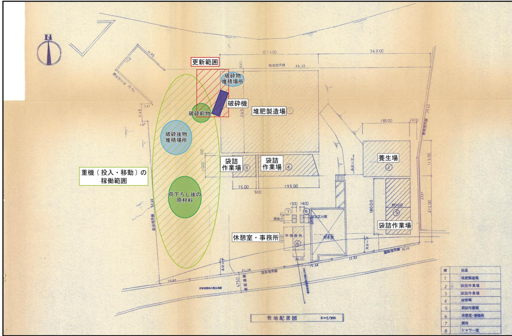
図 1-3 施設の主要設備配置図
